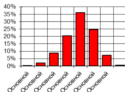
Рис.2. Гистограмма распределения длительностей R-R интервалов.
