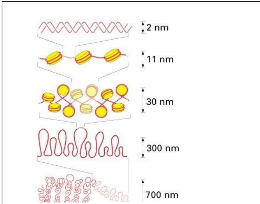
Рис. 2. Уровни компактизации
